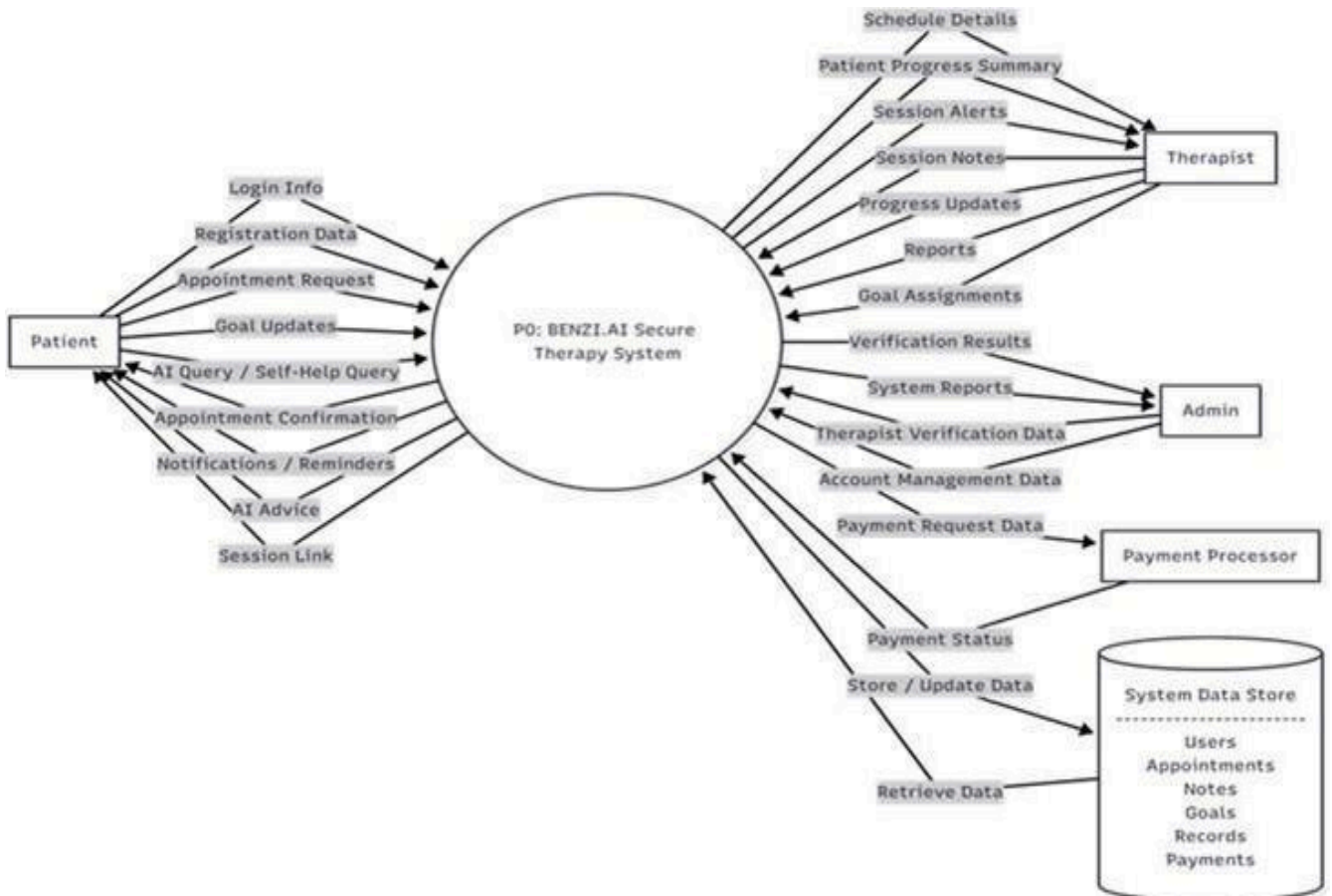
Fig 3.3 Level 0 DFD
