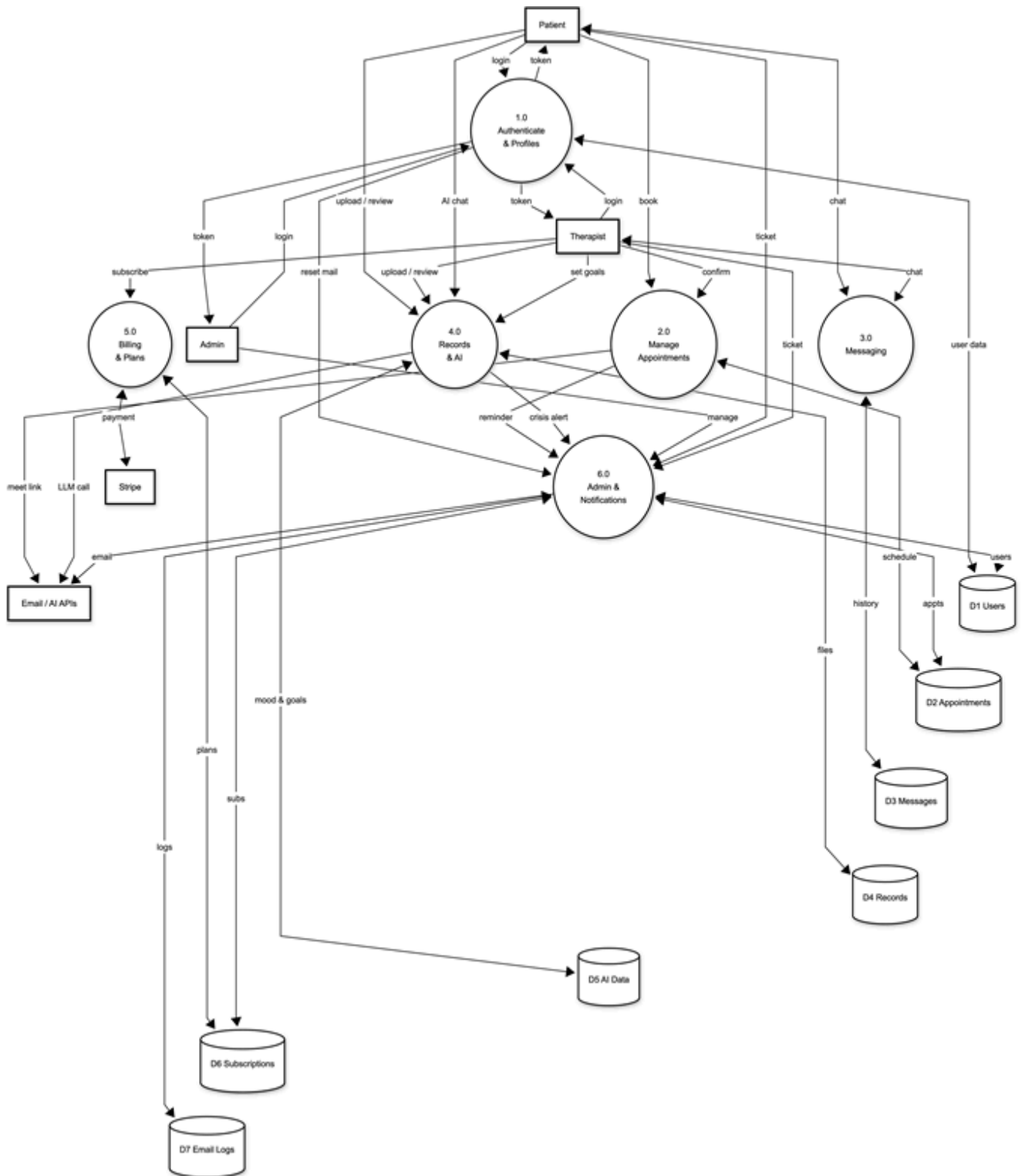
Fig 3.4 Level 1 DFD
